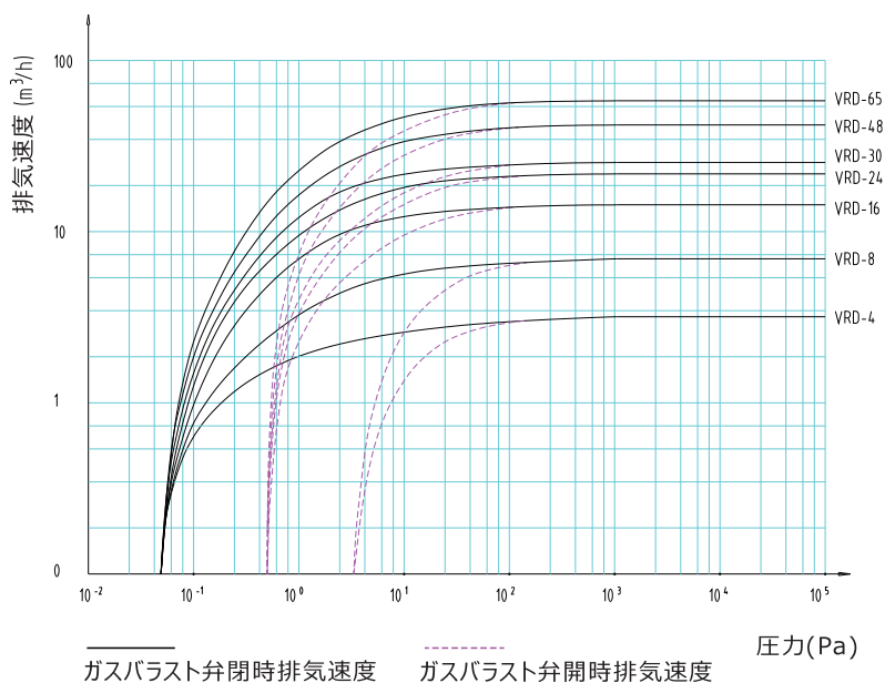
図 3 .排気速度曲線
