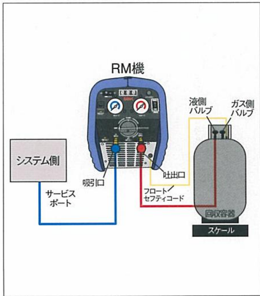
【液・ガス回収の接続図】
