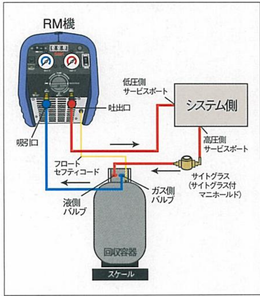
【プッシュプル回収の接続図】
